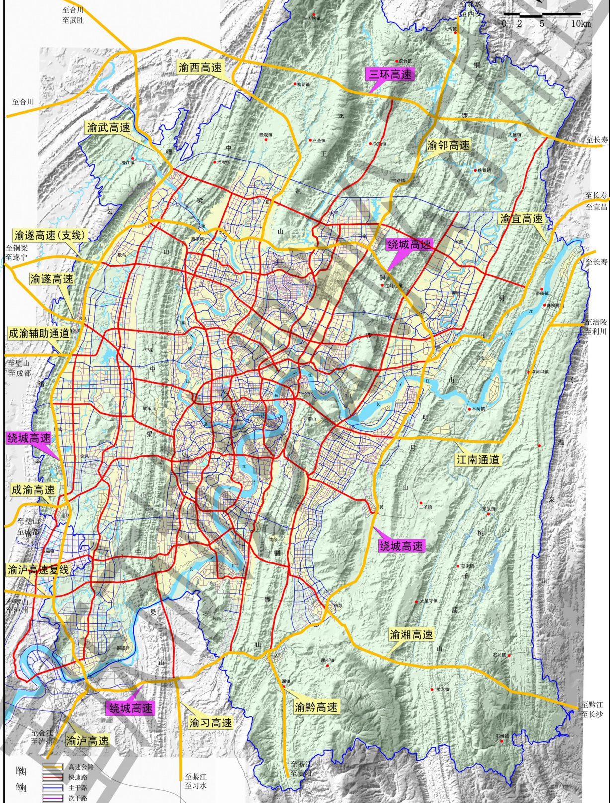
主城区道路网规划图
